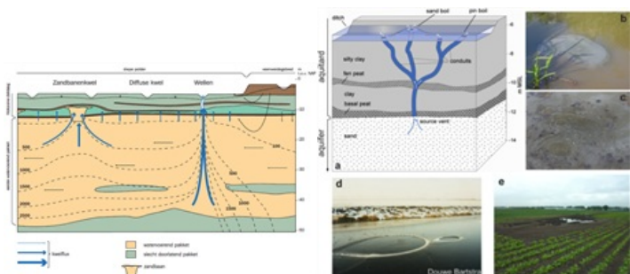
Fig. 2 Drie verschillende typen zoute kwel die verschillen in flux en zoutgehalte, schematische voorstelling van een wel in de deklaag en enkele foto's van wellen; (b) zandwel, (c) methaangas dat via wellen ontsnapt, (d) wellen en ijs, (e) een wel op het land (De Louw, 2013).
